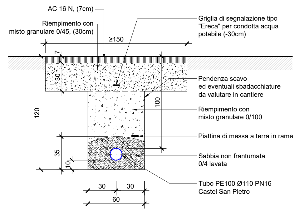
Sezione tipo posa 1:25
